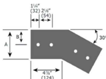
Éclisses 30° verticales
